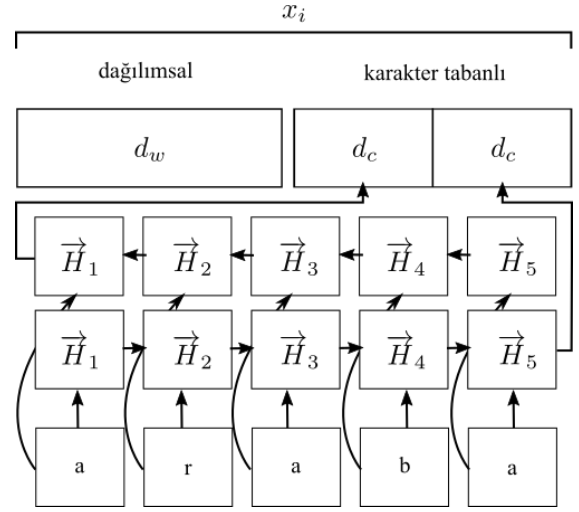
Şekil 1: Bi-LSTM kullanarak karakter tabanlı sözcük vektörünün oluşturulması. Ayrıca x_i sözcük vektörünün dağılımsal sözcük vektörüyle de ardarda eklendiği görülüyor.
